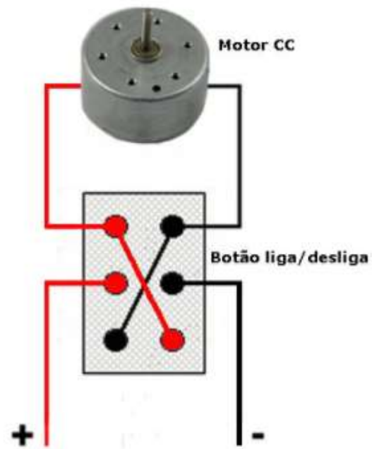
Figura 13: Esquema de ligação das botoeiras
