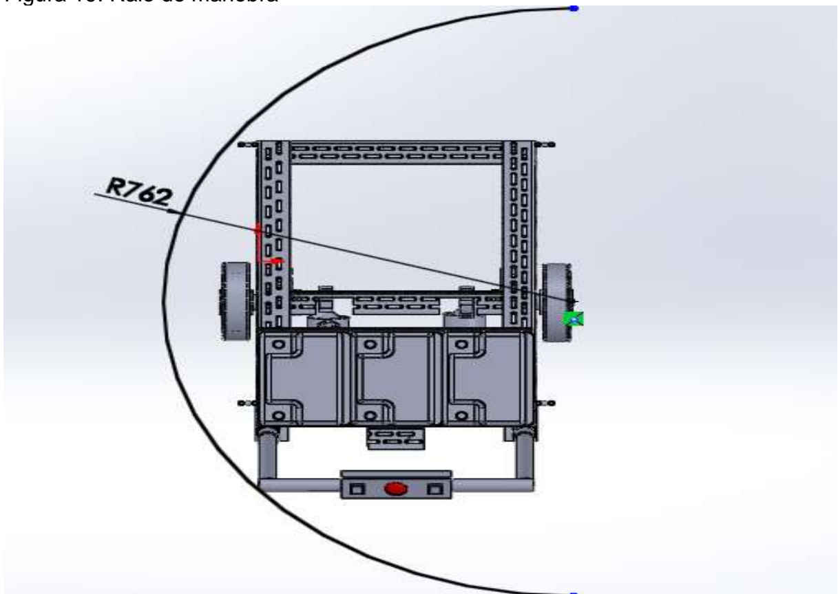
Figura 19: Raio de manobra
