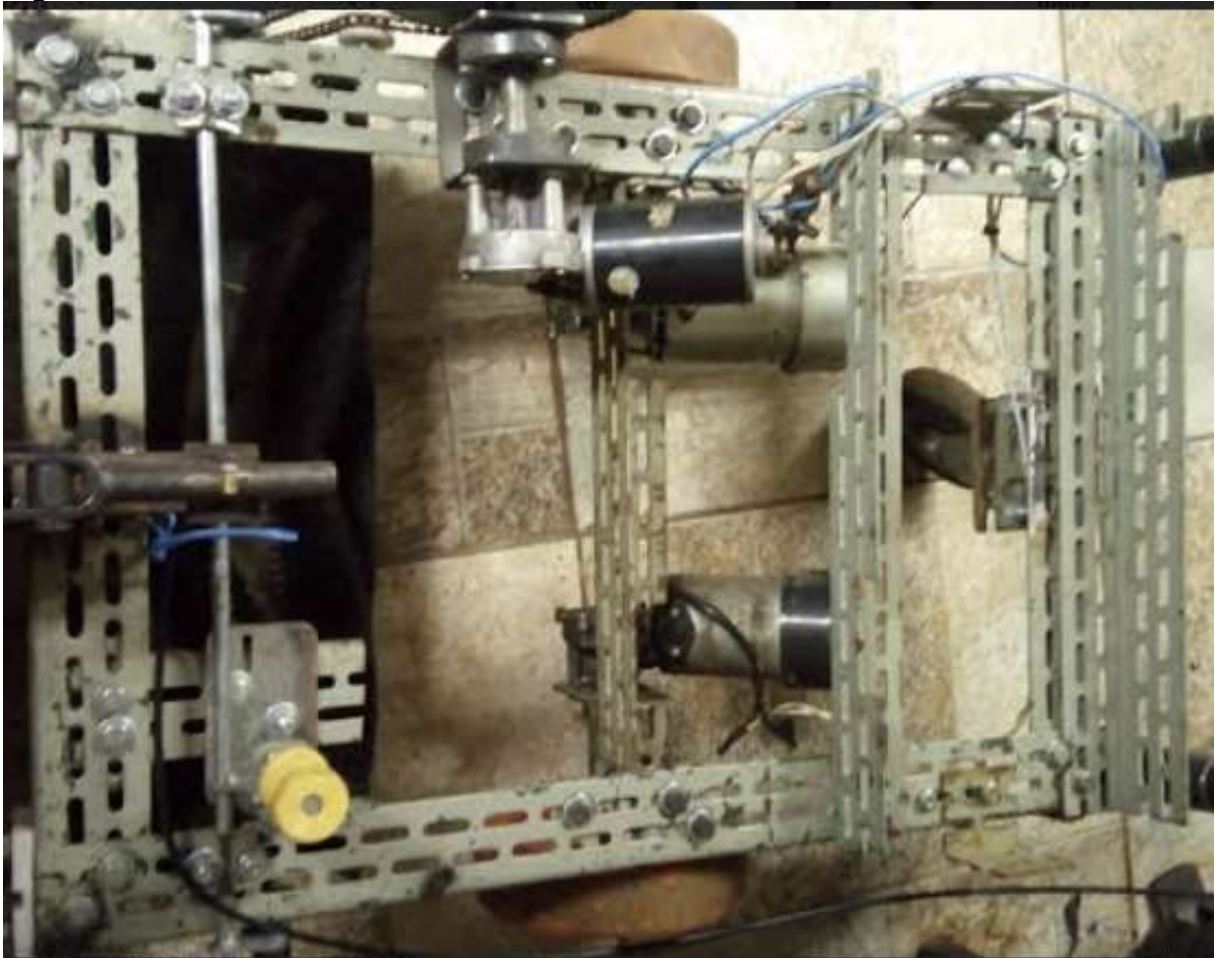
Figura 9: Chassi
