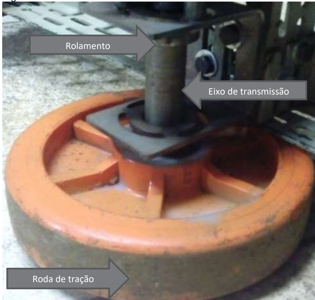
Figura 11: Sistema de transmissão
