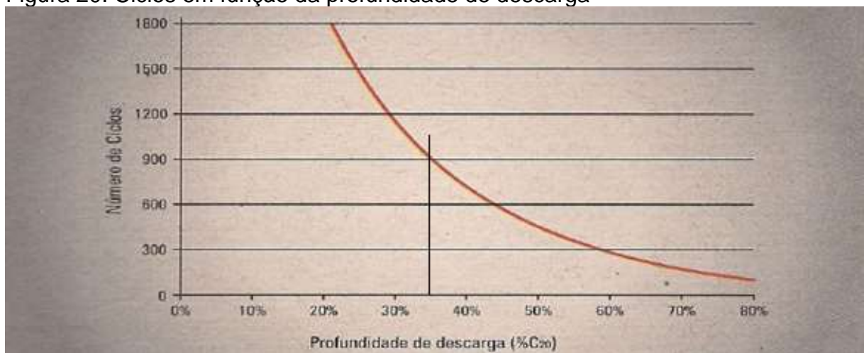
Figura 20: Ciclos em função da profundidade de descarga
