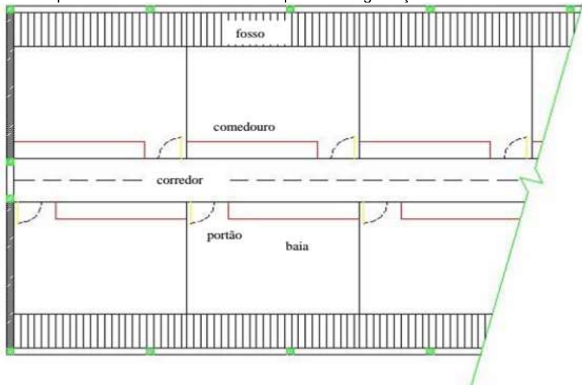
Figura 3: Esquema em planta baixa de um prédio com baias coletivas, possíveis de se usar para animais em crescimento e porcas em gestação
