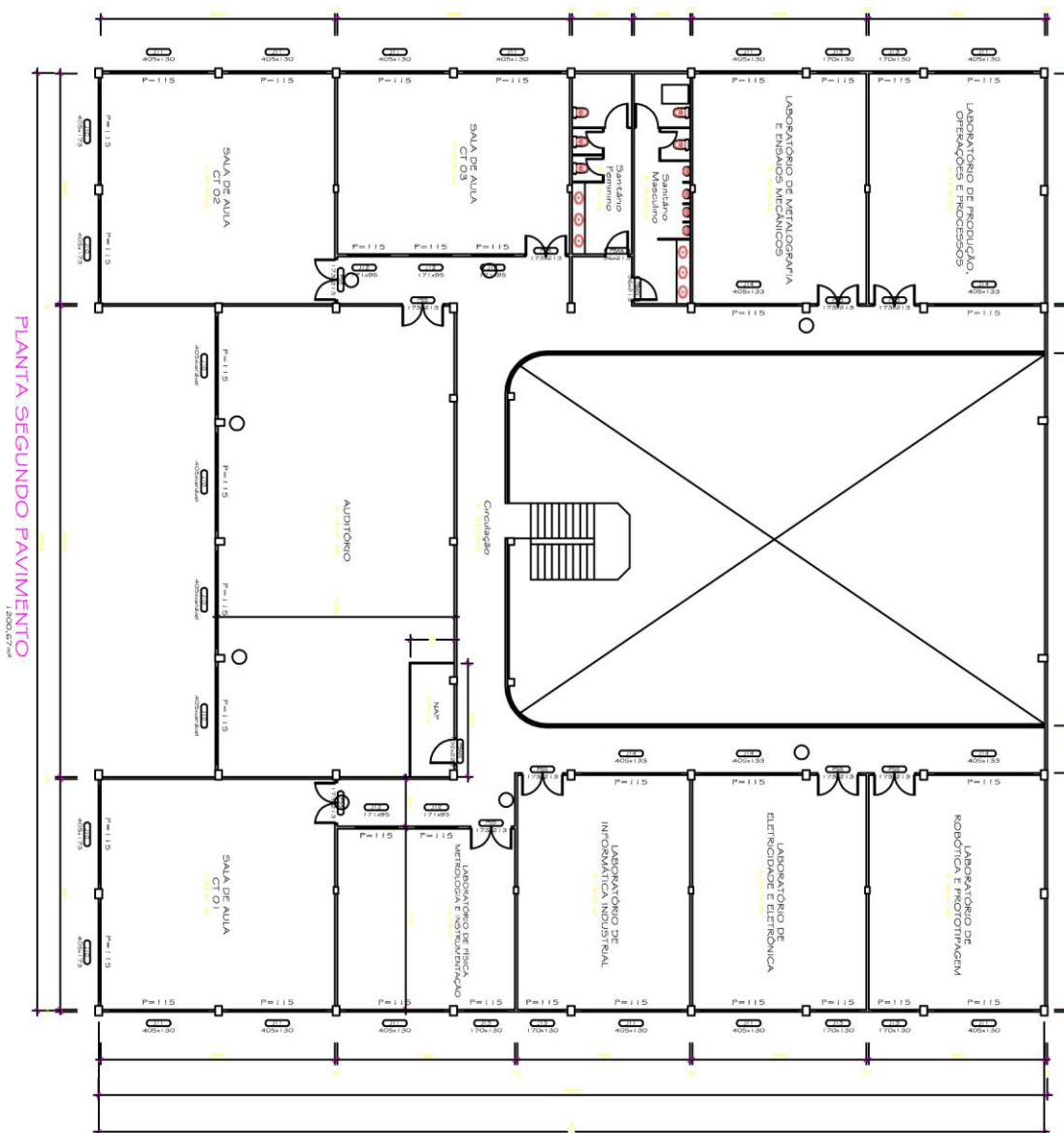
Figura 2. Segundo pavimento do Centro de Tecnologia.
